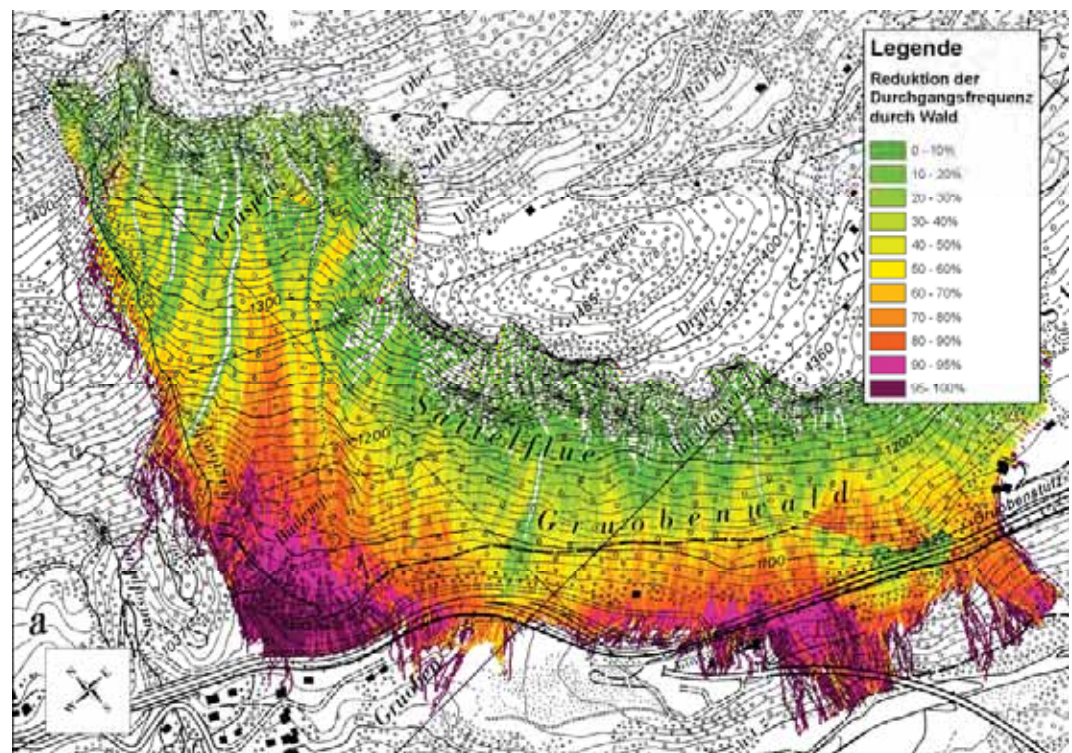
Abb. 12: Reduktion der Durchgangsfrequenz durch Wald: Reduktion der Durchgangsfrequenz durch „gepflegten Wald“ in Prozent zur Durchgangsfrequenz „ohne Wald“ für das häufige Szenario.
