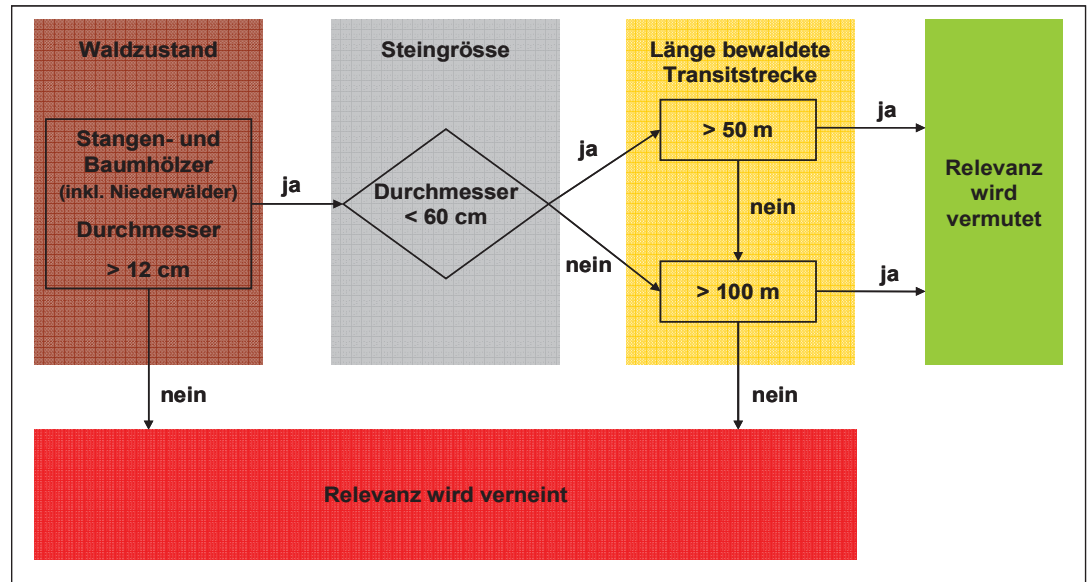
Abb. 5: angepasste Grobbeurteilung Sturz: In Abhängigkeit des Waldzustandes, der Steingrösse und der bewaldeten Transitstrecke wird die Relevanz von Schutzwäldern abgeschätzt.
