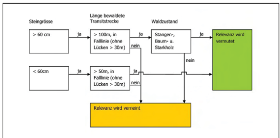
Abb. 4: Grobbeurteilung Sturz: Vorschlag für die Grobbeurteilung des Sturzprozesses aus Phase I.
