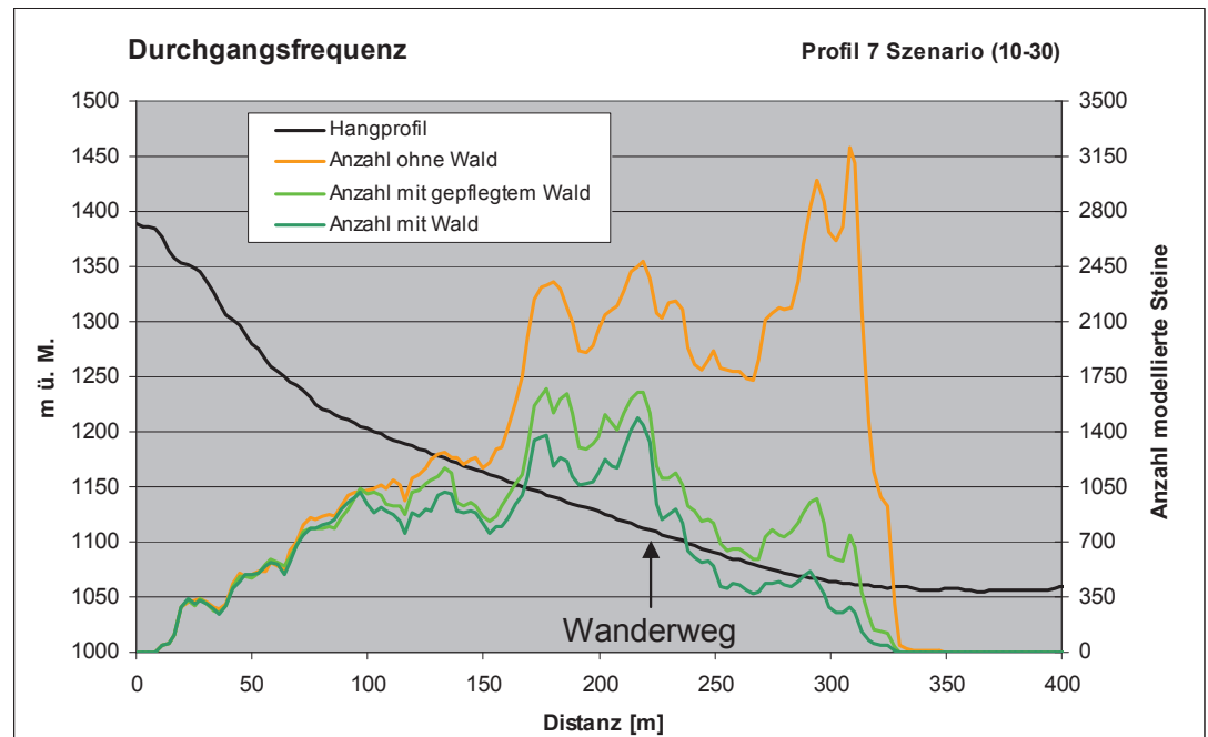
Abb. 14: Durchgangsfrequenzen: Bewaldet ist der Abschnitt zwischen 75 m und 315 m. Durch Wald wird die Durchgangsfrequenz stark reduziert. Wie im Feld zu beobachten, werden auch im Modell viele Steine auf dem Wanderweg abgelagert. (Das Profil befindet sich in einer Mulde, deshalb nimmt die Anzahl der modellierten Steine auch unterhalb der Ausbruchgebiete zu. Die räumliche Modellierung berücksichtigt auch Steine, welche seitlich in die Mulde stürzen).
