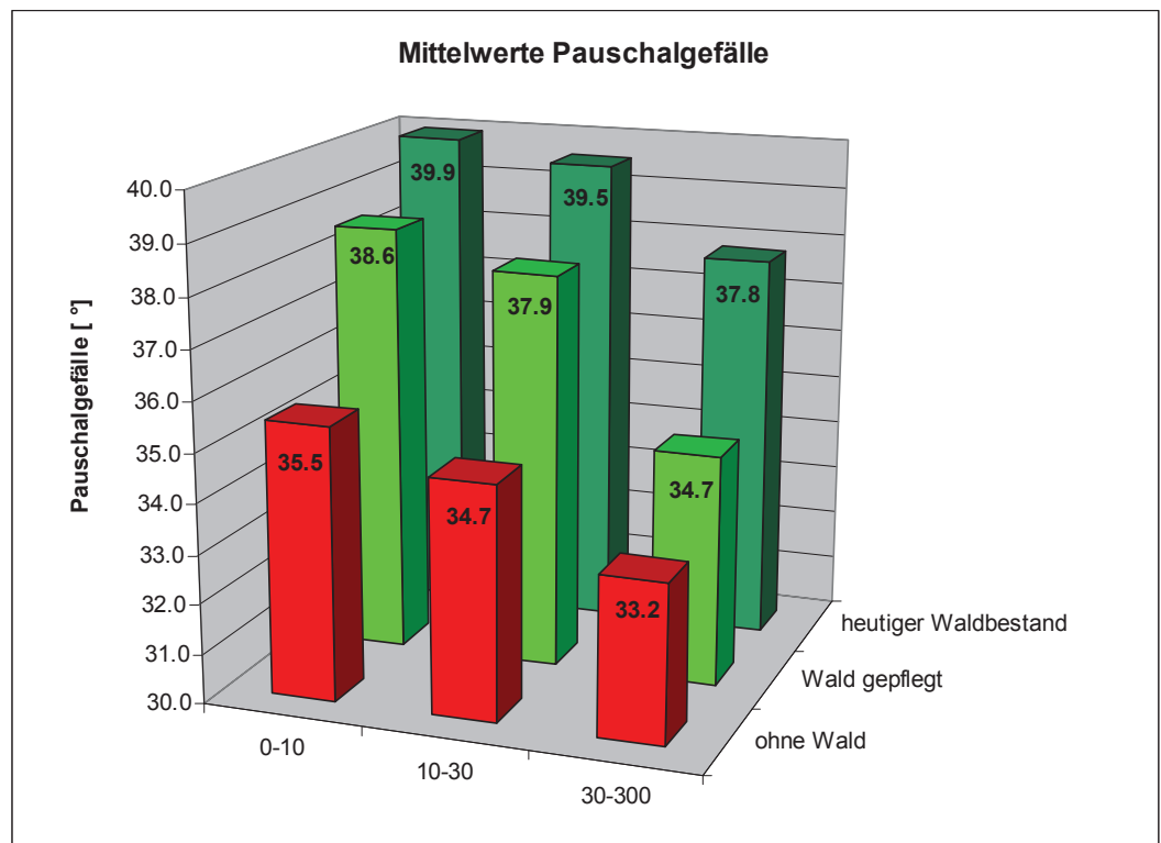
Abb. 10: Pauschalgefälle: Mittelwerte der Pauschalgefälle aller Szenarien. Das Pauschalgefälle bezeichnet den Winkel zwischen Ausbruchs- und Ablagerungsstelle.
