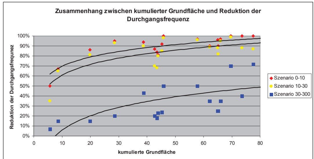
Abb. 16: Zusammenhang zwischen kumulierter Grundfläche und Reduktion der Durchgangsfrequenz: Die Wirkung des Waldes nimmt mit der kumulierten Grundfläche zu. Je grösser die modellierten Steine, desto geringer der Waldeinfluss auf die Reduktion der Durchgangsfrequenz.
