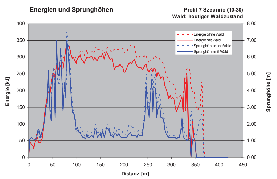
Abb. 13: Reduktion der Energie und Sprunghöhen durch Wald: Die maximalen Werte (95% Quantil) für die kinetische Energie und die Sprunghöhe werden durch Wald nur geringfügig reduziert. Bewaldet ist der Abschnitt zwischen 75 m und 315 m.
