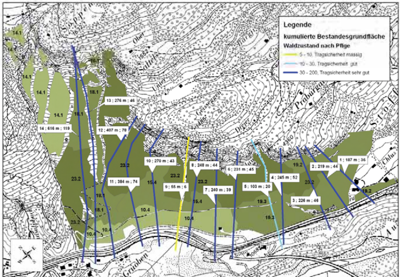
Abb. 7: Nachweis der Tragsicherheit: Auf Basis der Grundflächen der Bestände (schwarze Zahlen) wird entlang von Profilen die kumulierte Bestandesgrundfläche ermittelt. Angaben in den weissen Kästchen: Profilnummer, bewaldete Transitstrecke, kumulierte Bestandesgrundfläche.
