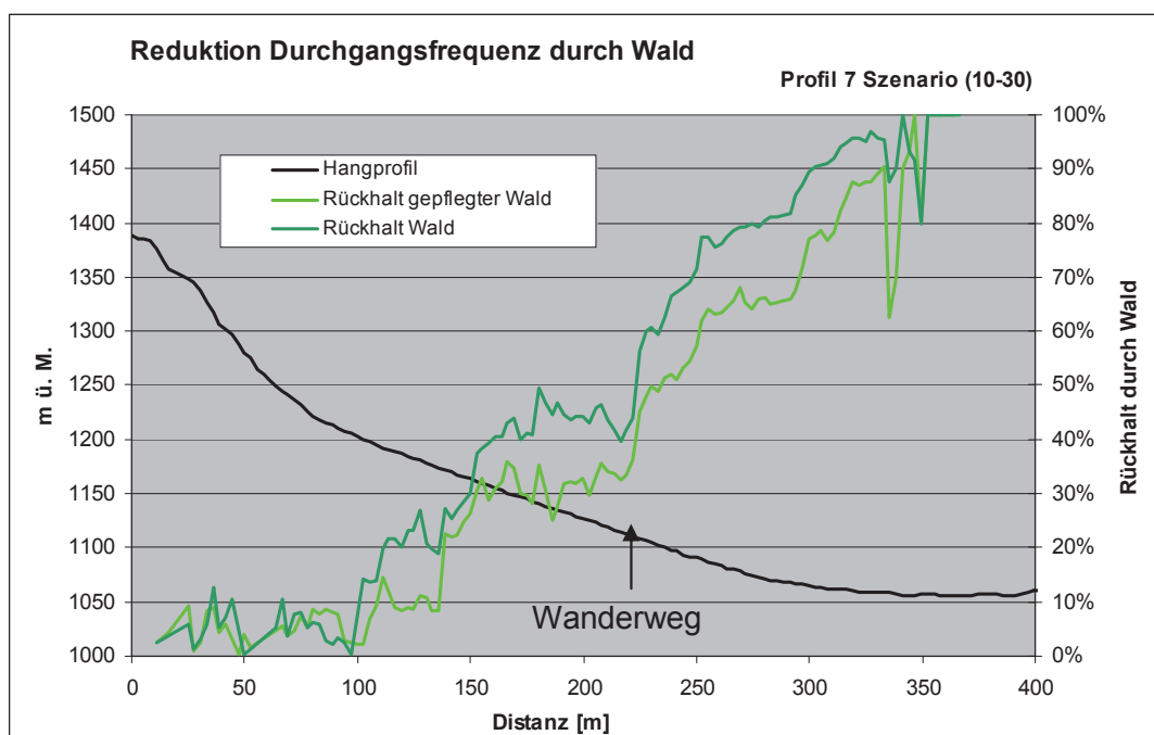
Abb. 15: Reduktion der Durchgangsfrequenz durch Wald: Reduktion der Durchgangsfrequenz durch Wald in Prozent zur Durchgangsfrequenz ohne Wald. Bewaldet ist der Abschnitt zwischen 75 m und 320 m.
