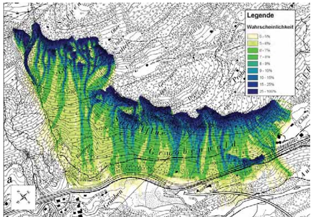
Abb. 11: Steinschlagaktivität: Modellerte Wahrscheinlichkeit von Steinschlag für das häufige Szenario ohne Wald. Je dunkler die Farben desto wahrscheinlicher ist das Auftreten von Steinschlag.
