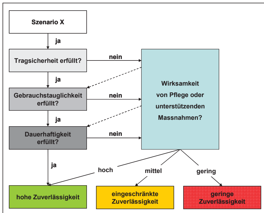
Abb. 6: Massnahmenbeurteilung: Die Massnahmenbeurteilung erfolgt anhand der Tragsicherheit, der Gebrauchstauglichkeit und der Dauerhaftigkeit. Sind diese erfüllt, besitzt der Schutzwald eine hohe Zuverlässigkeit. Ist einer dieser Faktoren nicht erfüllt, hängt die Zuverlässigkeit von der Wirksamkeit der Pflege oder unterstützenden Massnahmen ab.
